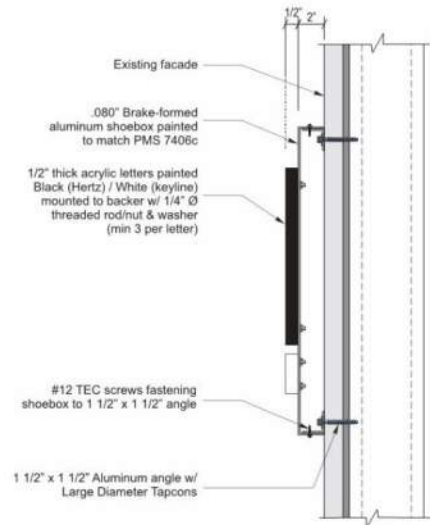
Section @ Non-Illuminated Letters Scale: N.T.S.
